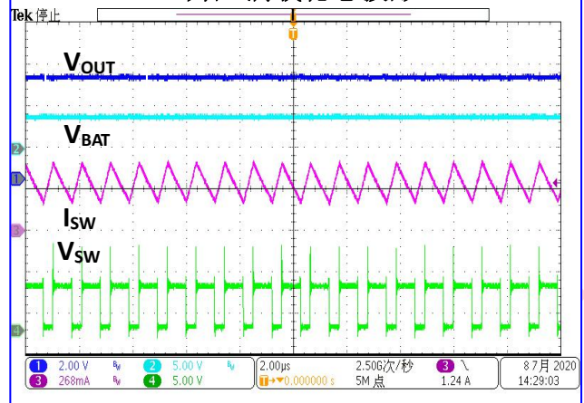
升压满载稳态波形
