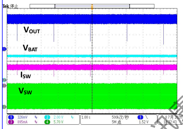
放电模式 VBUS 检测周期
