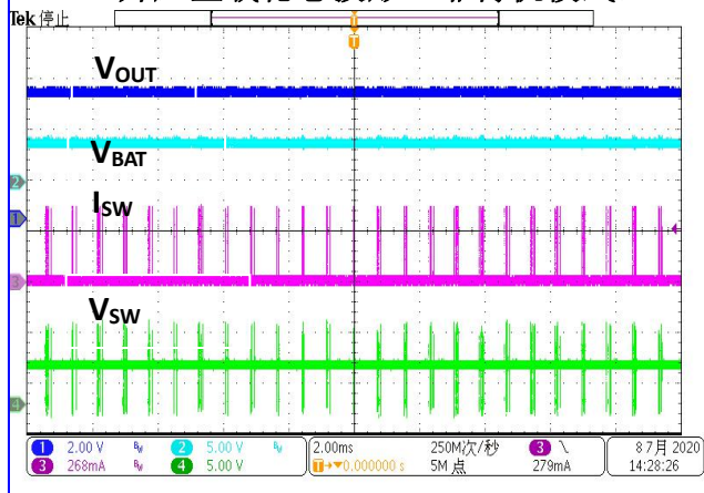
升压空载稳态波形（非待机模式）
