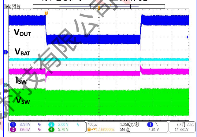
放电模式 VBUS 检测脉宽
