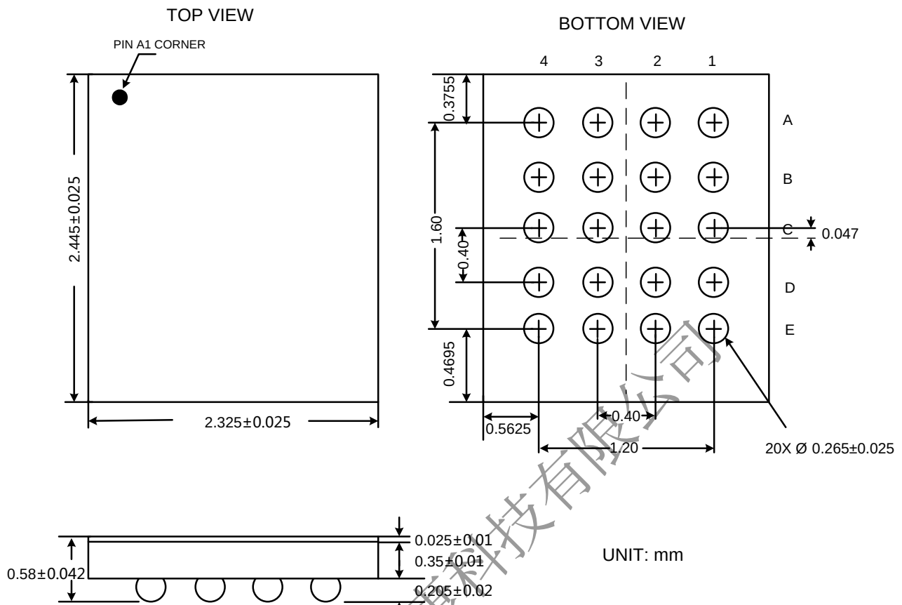
图 31 NS2158 WCSP 封装信息
