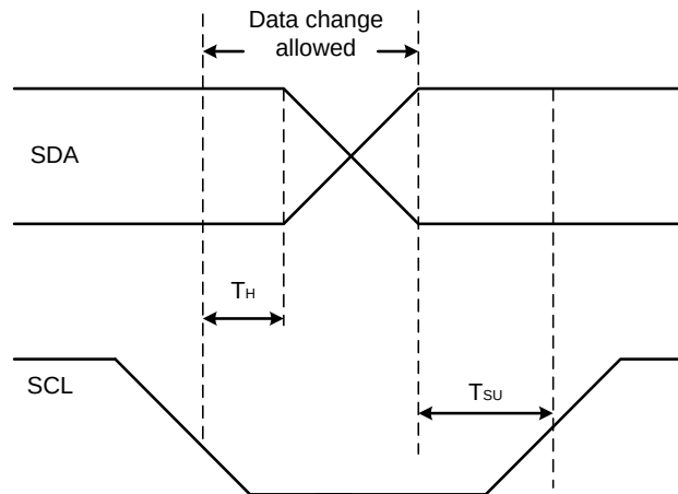
图 21 I 2 C 数据传输规则
