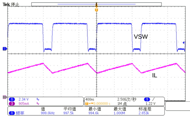
图 3 V_{\text{BUS}}=5\text{V} , V_{\text{BAT}}=3.8\text{V} , I_{\text{O(CHAARGE)}}=2.16\text{A} , PWM 充电波形
