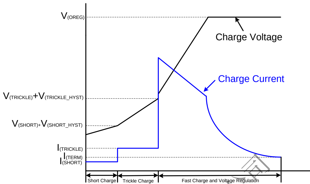
图 18 NS2158 Input Current Limit 充电流程图
