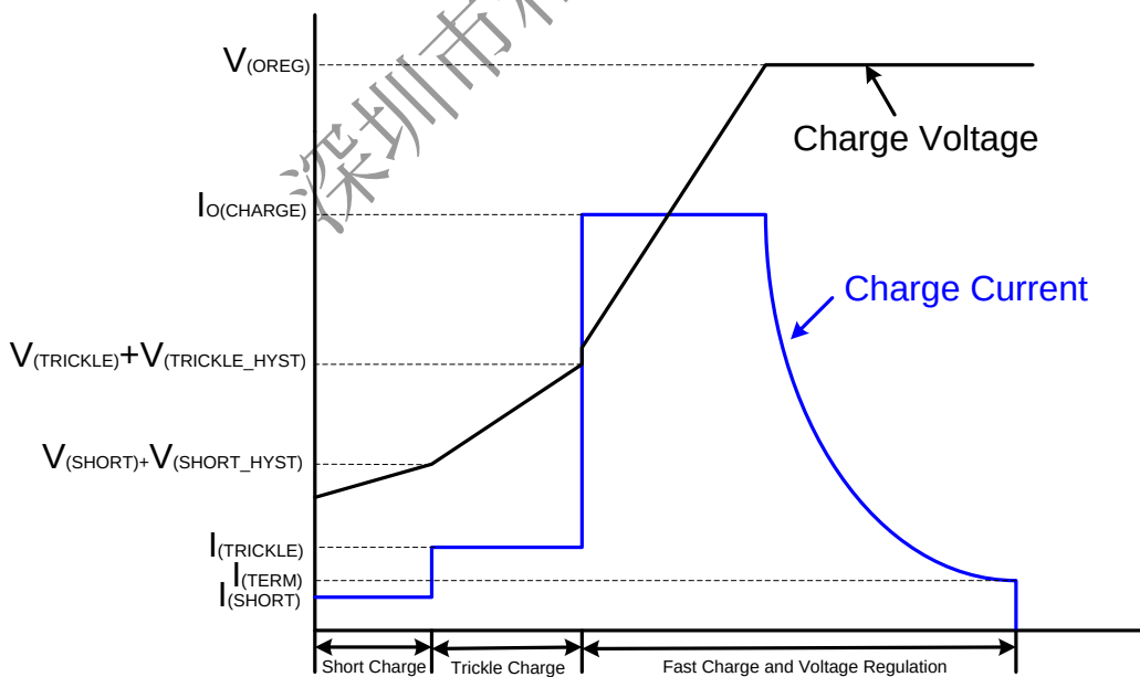
图 17 NS2158 Without Input Current Limit 充电流程图
