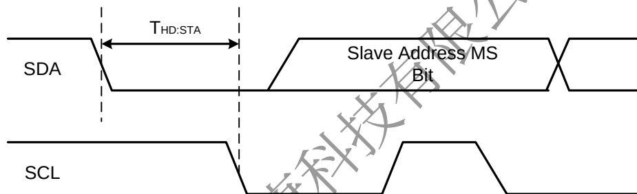
图 22 I 2 C 起始条件
