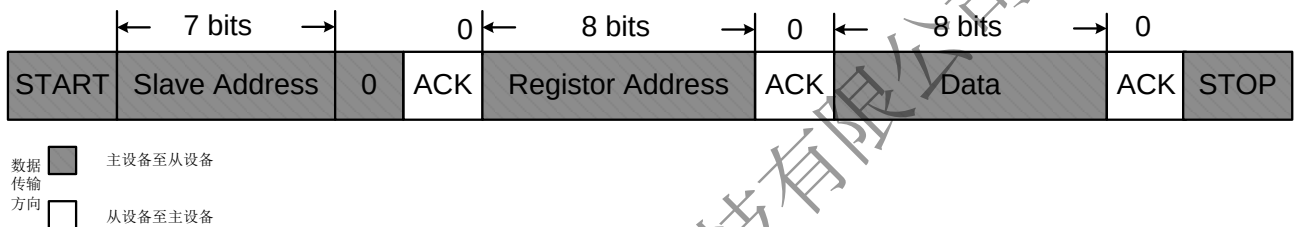
图 25 I 2 C 写操作
