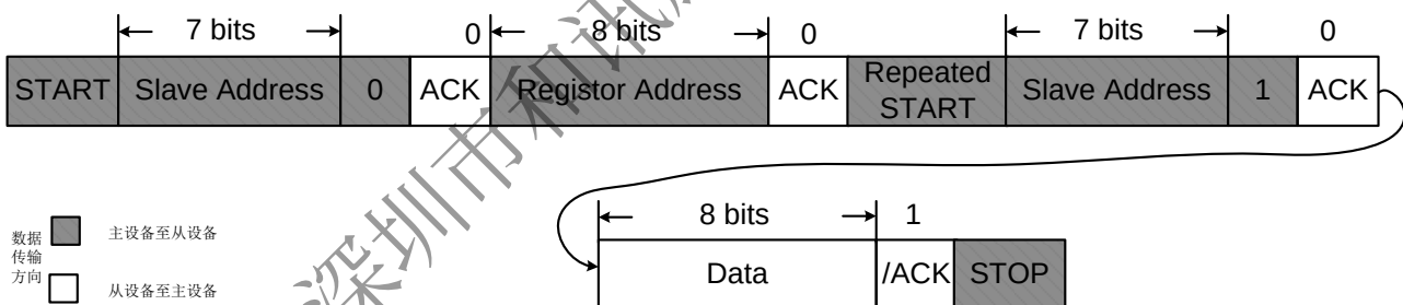
图 26 I 2 C 读操作
