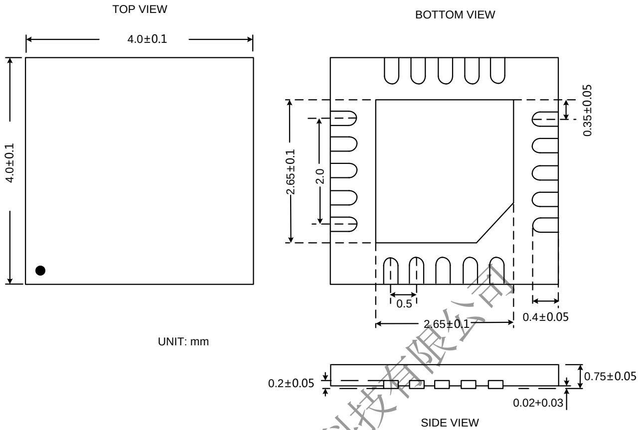
图 32 NS2158 QFN 封装信息
