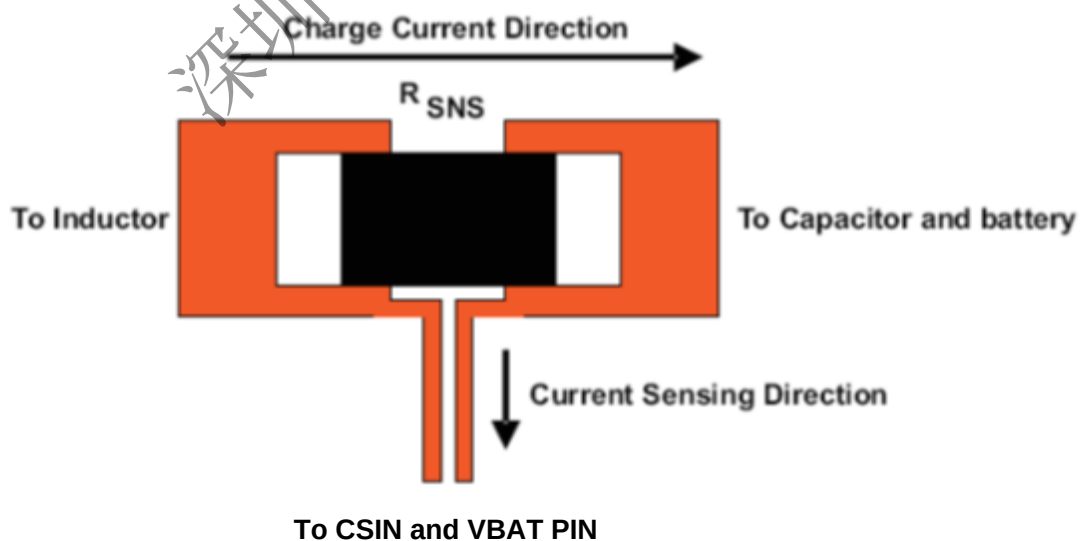
图 29 RSNS 电阻 PCB Layout 举例
