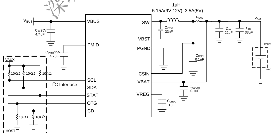
图 1 NS2158 典型应用电路
