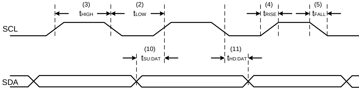
图 19 SCL 与 SDA 在数据传输过程中的时序关系
