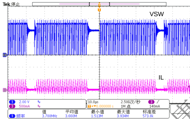
图 11 OTG 模式, V_{BAT}=4V , I_{LOAD}=50mA , PFM 模式
