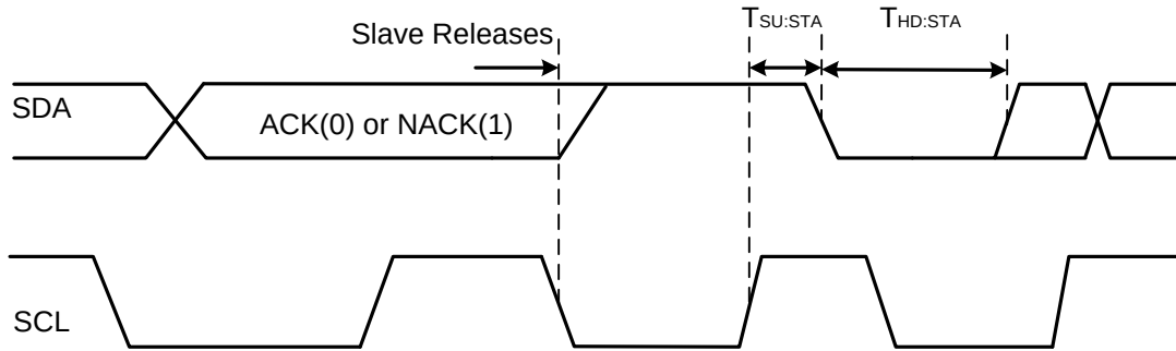
图 24 I 2 C 重复起始
