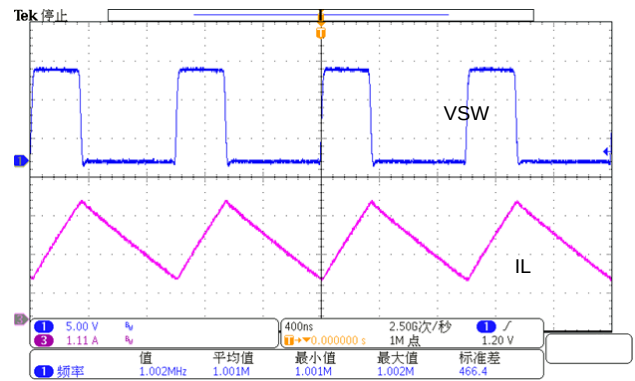
图 4 V_{\text{BUS}}=12\text{V} , V_{\text{BAT}}=3.8\text{V} , I_{\text{O(CHAARGE)}}=2.16\text{A} , PWM 充电波形
