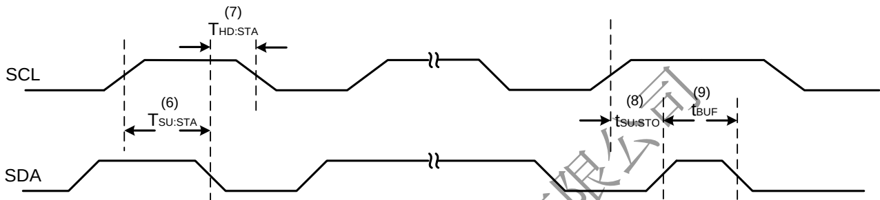
图 20 START 状态与 STOP 状态的时序关系
