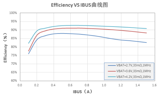
图 15 OTG 模式, OTG Efficiency vs. I_{OUT}
