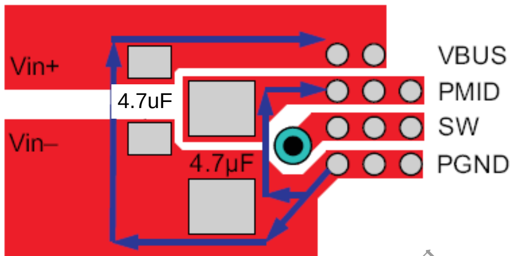
图 30 输入电容位置和 PCB layout 举例
