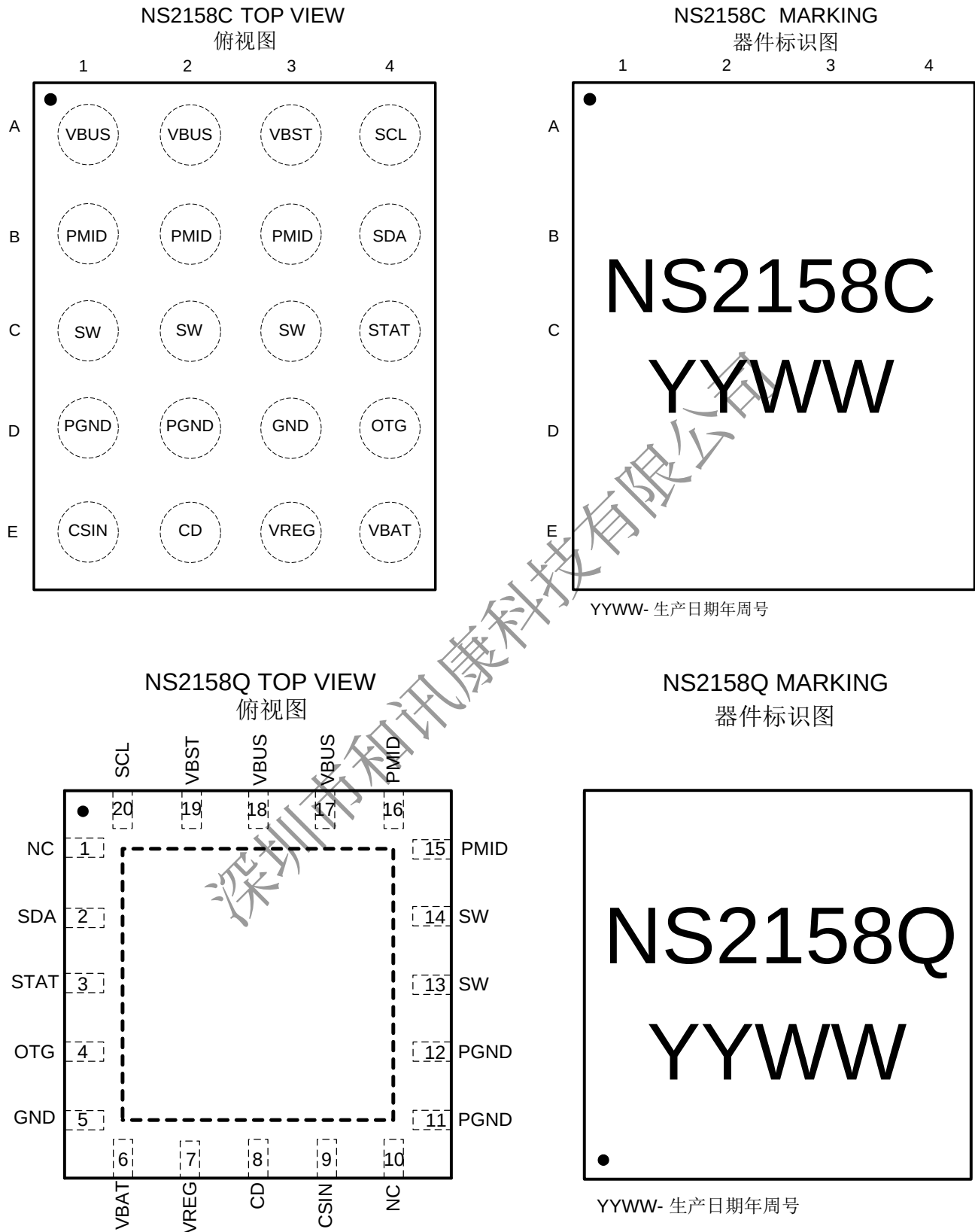
图 2 NS2158 引脚分布俯视图和器件标识图
