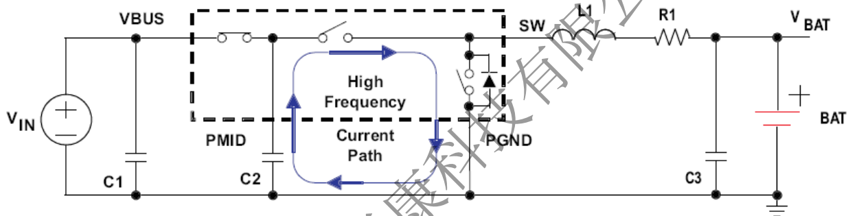
图 28 高频电流环路路径
