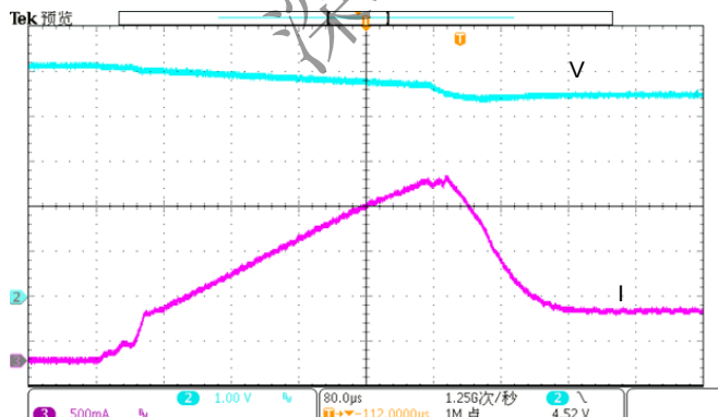
图 7 V_{\text{BUS}}=5\text{V} 限流 500mA, V_{\text{BAT}}=3.8\text{V} , I_{\text{O(CHAARGE)}}=2.164\text{A} , V_{\text{IN\_DPM}}=4.52\text{V} , V_{\text{IN\_DPM}} 响应
