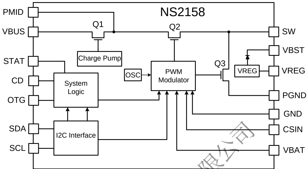
图 16 NS2158 功能结构框图
