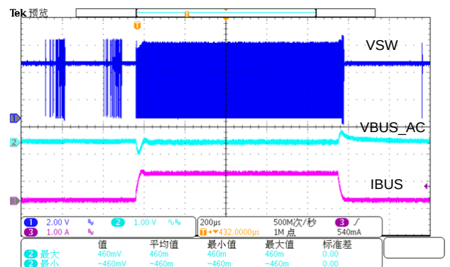
图 14 OTG 模式, Load Regulation, I_{LOAD} 0-1A-0, V_{BAT}=4V , t_f, t_r < 100ns
