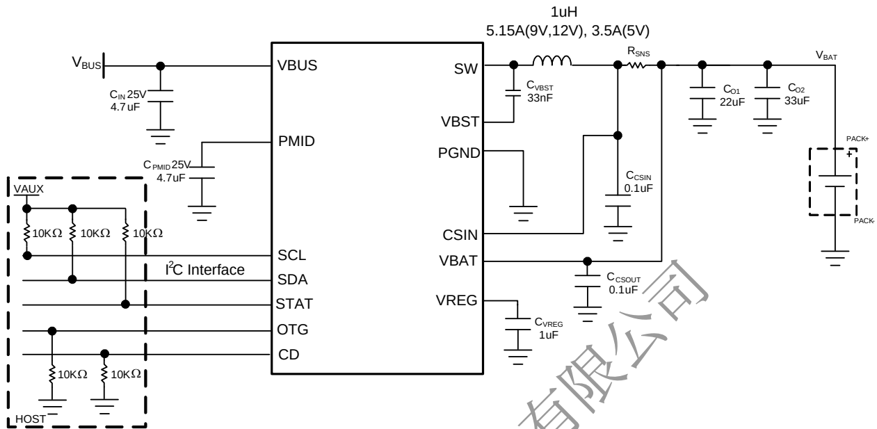
图 27 NS2158 典型应用电路
